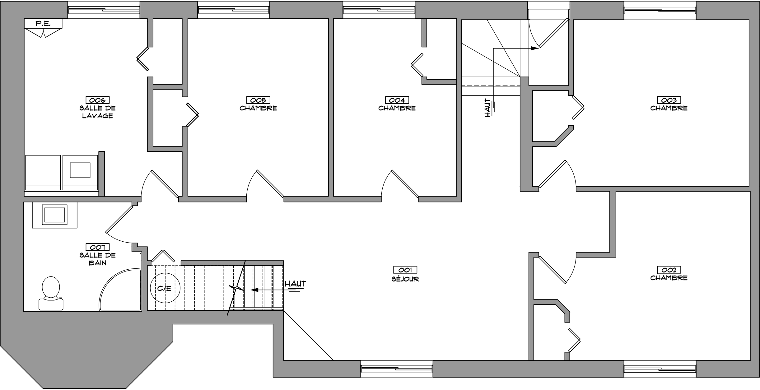
PLAN DU SOUS-SOL
